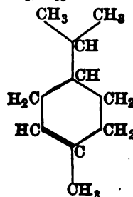
Carvomenthene.
